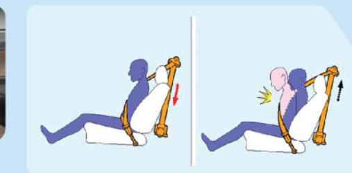
Front Seat Belt with Pretensioner & Force Limiter Seat Belt dirancang khusus untuk mengurangi potensi cedera saat airbag mengembang
